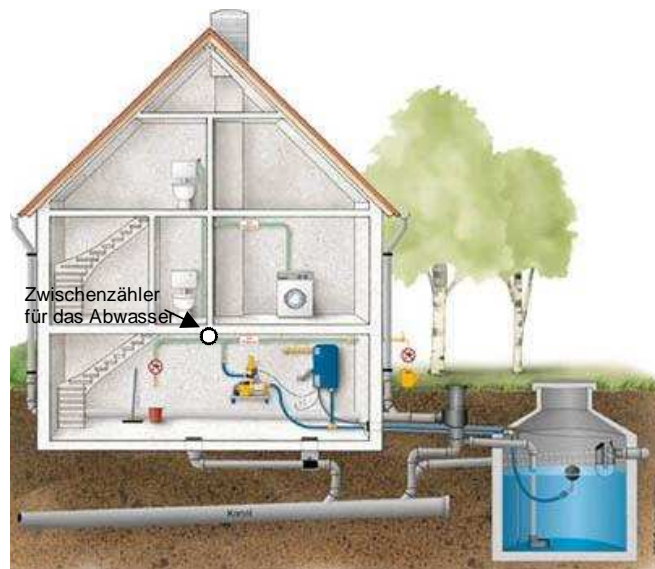
Skizze: Einbauort des Zwischenzählers vor den Verbrauchern
